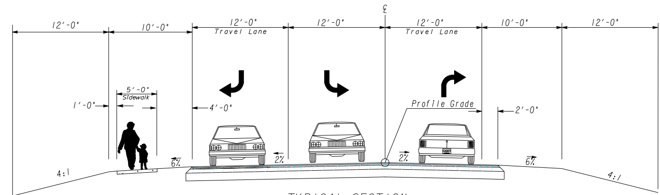
TYPICAL SECTION N. T. S.
